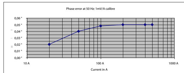
Phase shift
