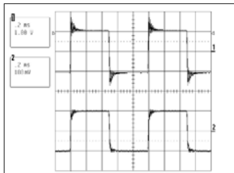
200 A calibre
