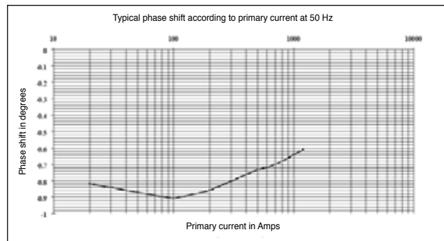
Phase shift
